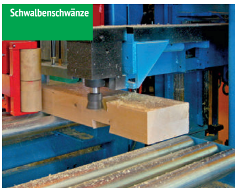
Schwalbenschwanz am Schifter
