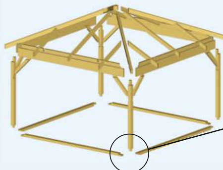
Detail Ecküberblattung mit Zapfen Abb. Konstruktion mit Fundamentrahmen
