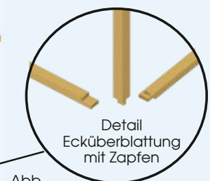
Detail Ecküberblattung mit Zapfen Abb. Konstruktion mit Fundamentrahmen
